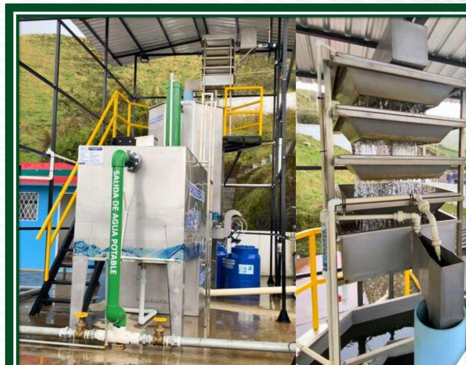
Planta de Agua Potable Tisaleo
